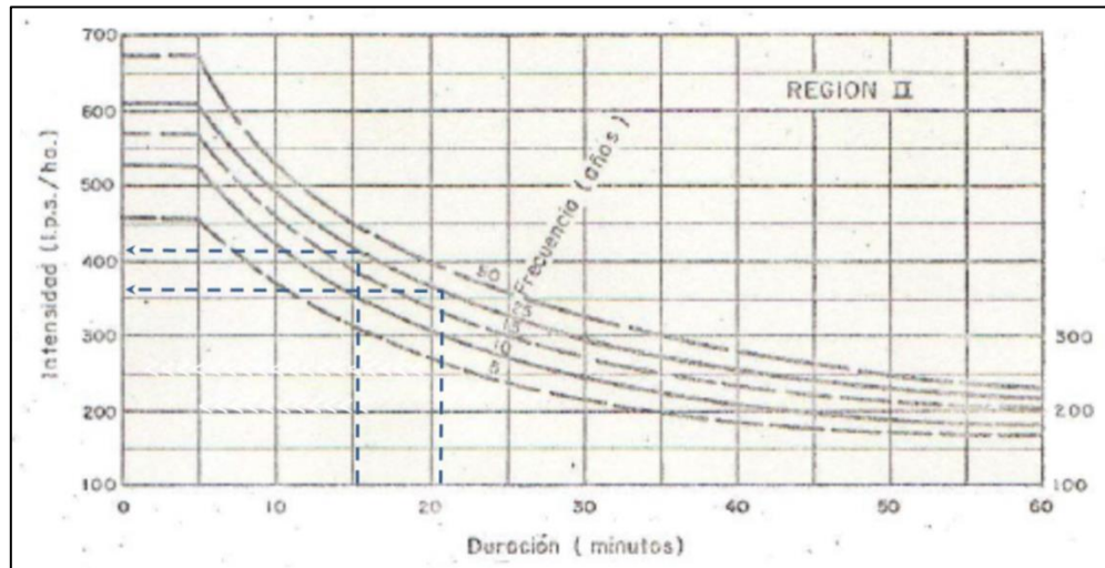
Figura 5.8 Curvas IDF de la Región Hidrológica II (MOP, 1967).
