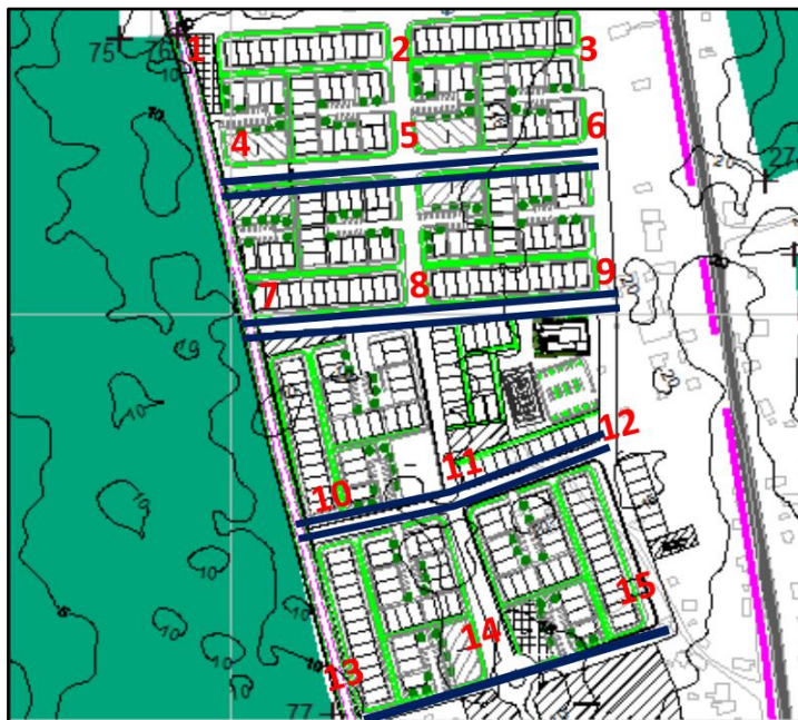
Figura 5.9 Trazado en planta de los canales principales del sistema de drenaje.
