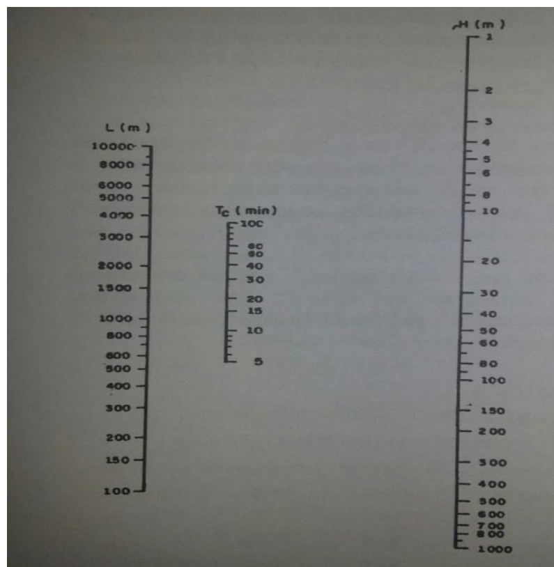
Figura 3.1. Abaco para estimación del tiempo de concentración en cuencas rurales (Arocha, 2012).
