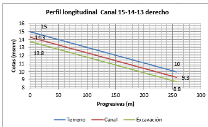
Figura 5.13 Perfil longitudinal del canal 15-14-13 derecho de la sub-cuenca verde.
