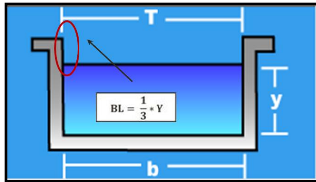
Figura 6.3 Sección transversal rectangular tipo de los canales propuestos.
