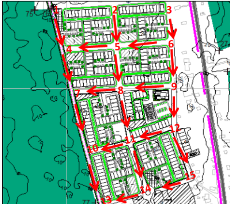
Figura 5.6 Códigos de parcelas y líneas de flujo del área de estudio: Este (amarilla) y Oeste (azul).
