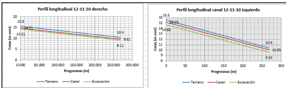
Figura 5.12 Perfiles longitudinales de los canales 12-11-10 derecho e izquierdo de la sub-cuenca roja.
