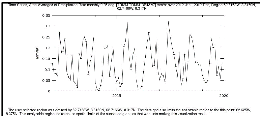
Figura 5.4 Rata de precipitación mensual en mm/hr. Período 2012 – 2019. Área Puerto Ordaz (servidor Giovanni)
