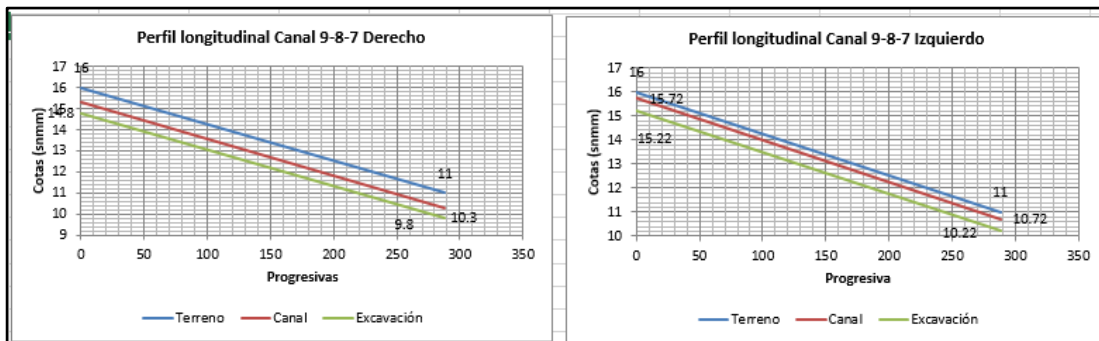
Figura 5.11 Perfiles longitudinales de los canales 9-8-7 derecho e izquierdo de la sub-cuenca amarilla.
