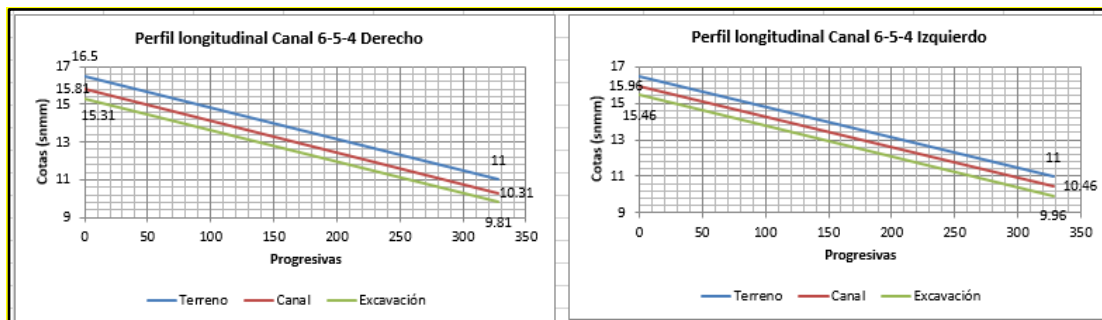
Figura 5.10 Perfiles longitudinales de los canales 6-5-4 derecho e izquierdo de la subcuena azul.
